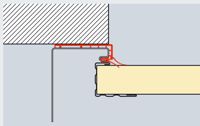
Mocowanie boczne z zastosowaniem ThermoFrame
