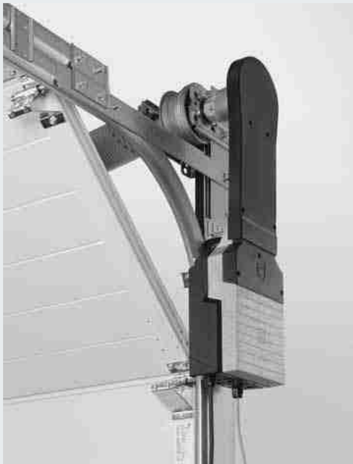
Pionowy wariant montażowy
