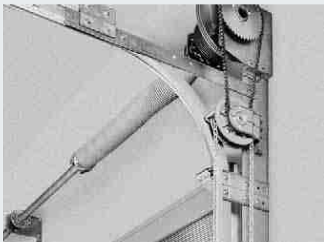
Opcjonalnie: napęd ręczny z przekładnią łańcuchową
