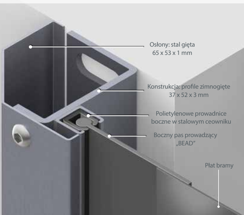
Prowadnice boczne z technologią „Low friction”
